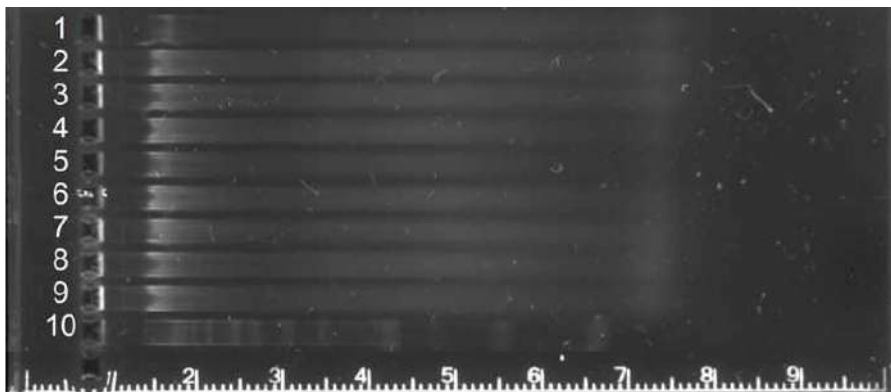
Рисунок 4 – Электрофореграмма ДНК различных сортов салата посевого, выделенной методом с SDS в трех повторностях: 1-3 – Афицион, 4-6 – Роксай, 7-9 – Фриллис, 10 – ДНК маркер Sky-High
